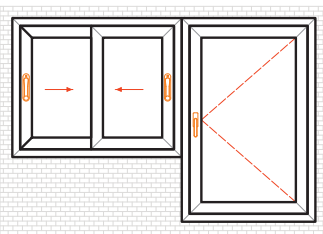
DOOR CUM WINDOW
